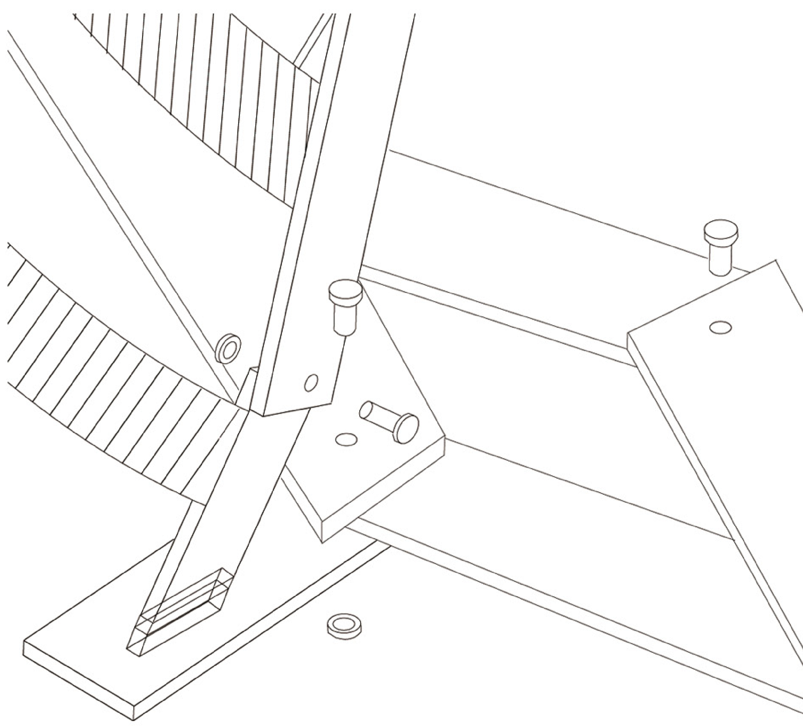
detalle constructivo del modelo abstracto que representa el movimiento estudiado.
