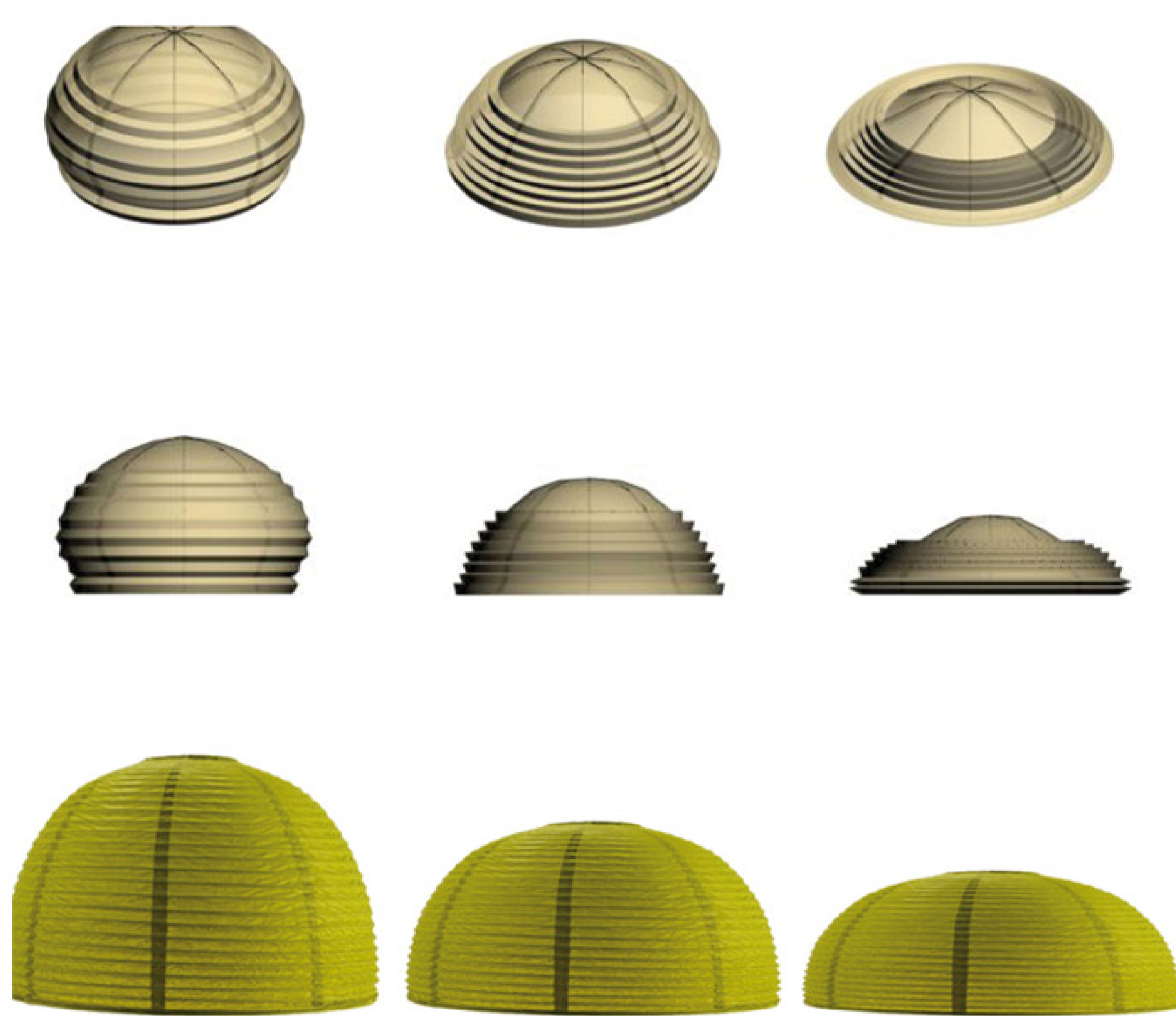
modelo y fotografía de la piel estudiada y propuesta.
